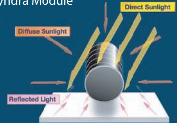
Solyndra Module
